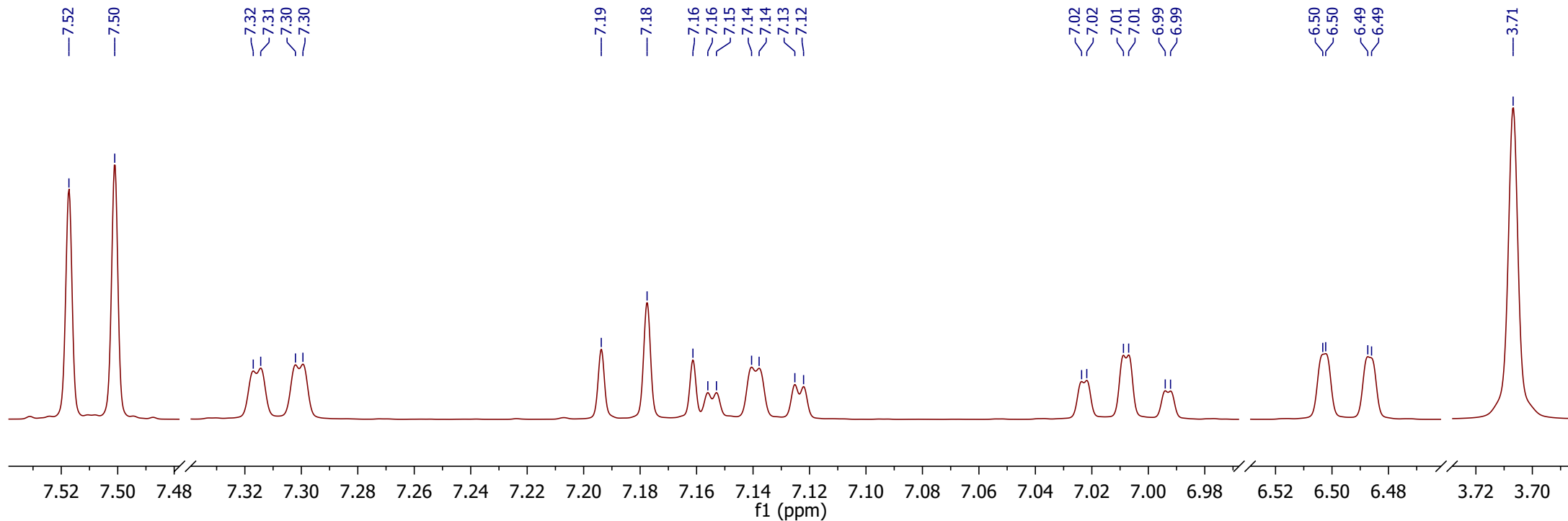
DCF_proton_vyrez_spektra_duraz_na_rozliseni
