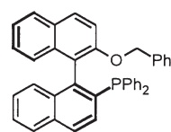
(S)-(-)-VI (cit. 3 )
