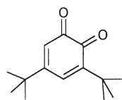
DTBBQ
