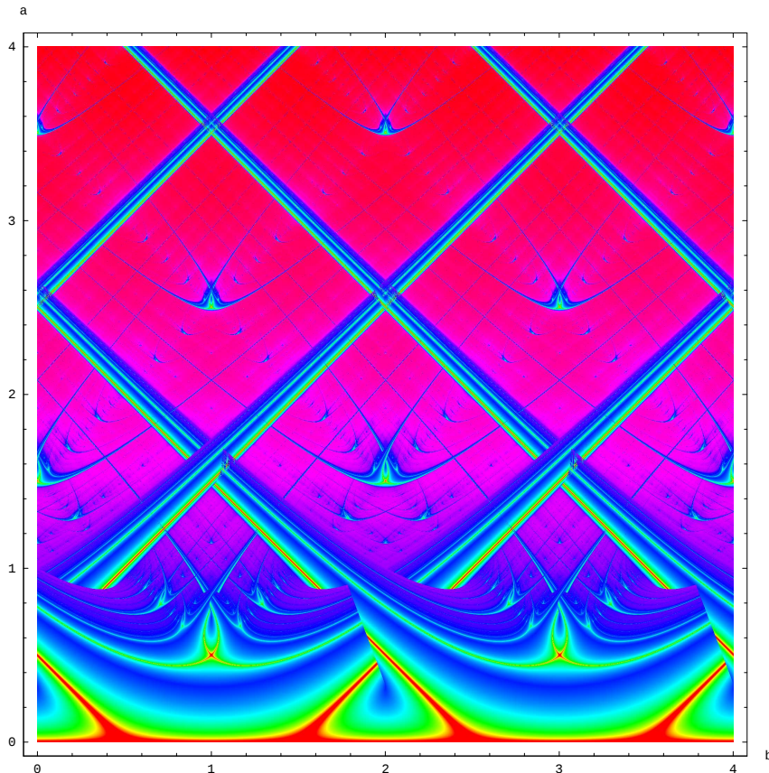
Obr. 4: Závislost Lyapunovova exponentu systému (5) na parametrech a a b .
