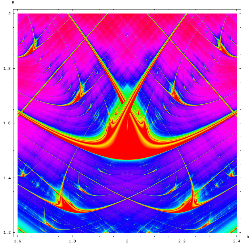
Obr. 5: Výřez z obrázku 4 ukazující fraktální strukturu v parametrickém prostoru.
