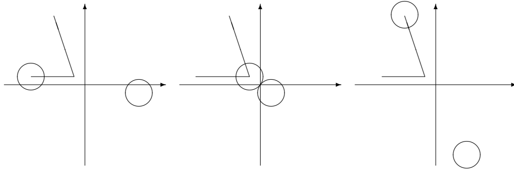
Obr. 2: Dvě molekuly (a) před srážkou, (b) při srážce, (c) po srážce.
