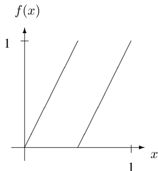
Obr. 1: Bernoulliho shift představuje elementární příklad systému s hustou množinou periodických bodů a také elementární příklad deterministického chaosu.
